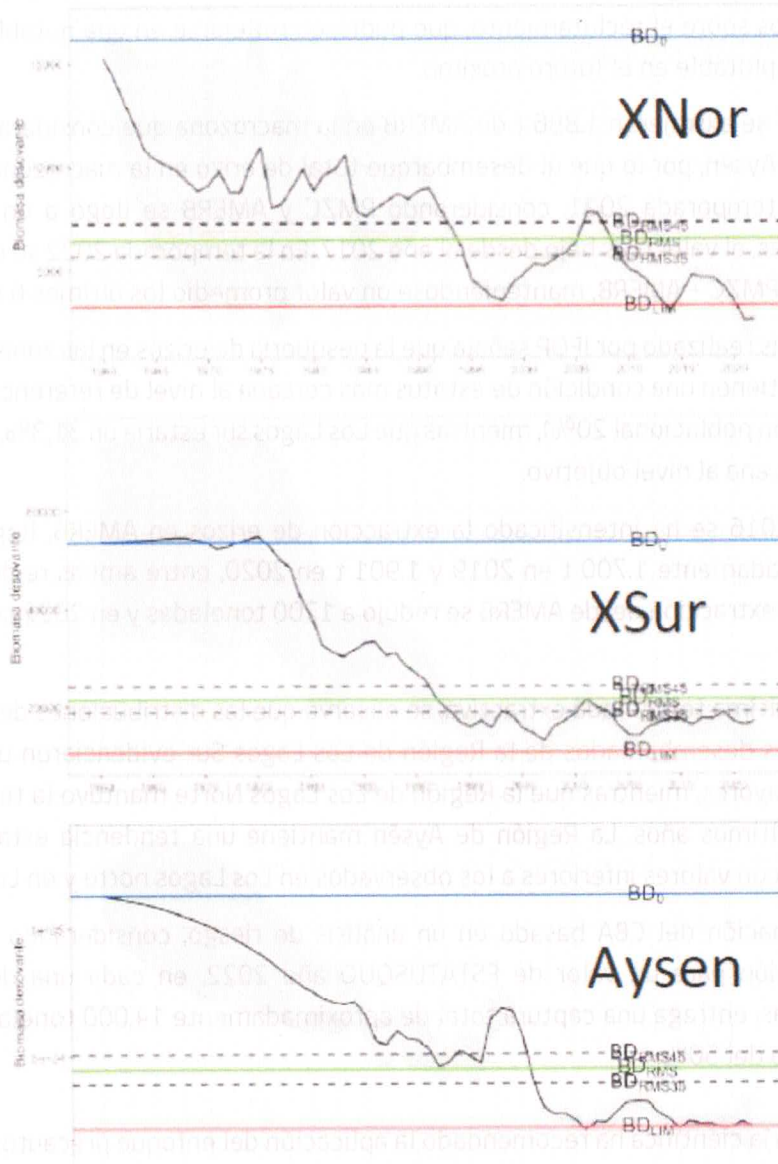
Figura 3. Modelado de biomasa desovante de erizo, obtenidas por el modelo base, por zona (X Nor, X Sur y Aysén), para las Regiones de Los Lagos y Aysén. Se señala una banda de PBR de 35%–45%, junto al de un 40% de agotamiento para BDo. Fuente: Programa de Seguimiento de Pesquerías Bentónicas bajo Régimen de Planes de Manejo.
