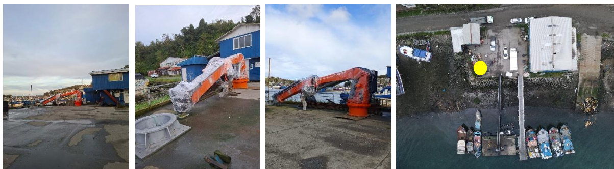
Figura N° 6: Vista Grúa instalada y punto de localización en la caleta (color amarillo)
